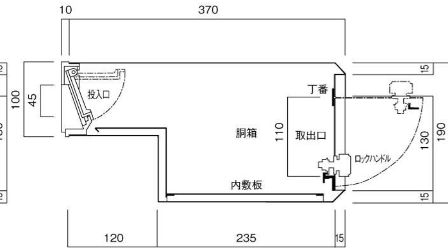
縦断面図
