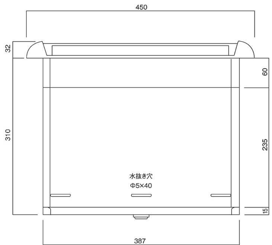
底面図
