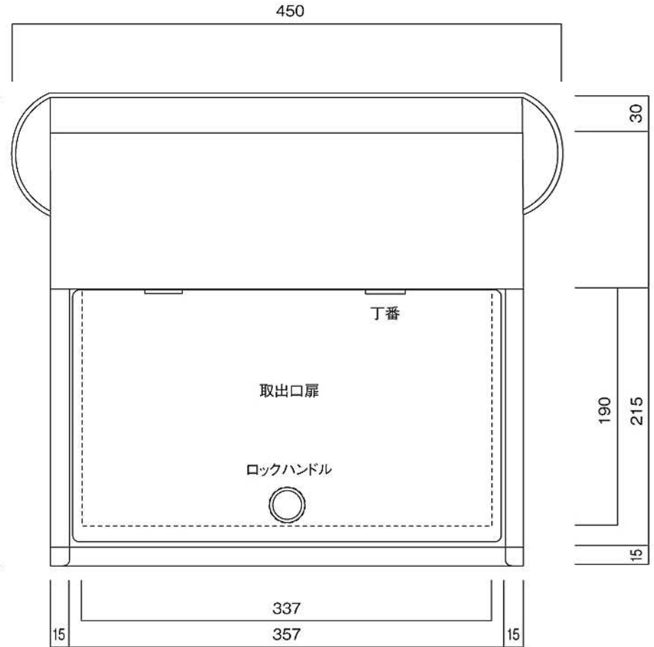
裏面図
