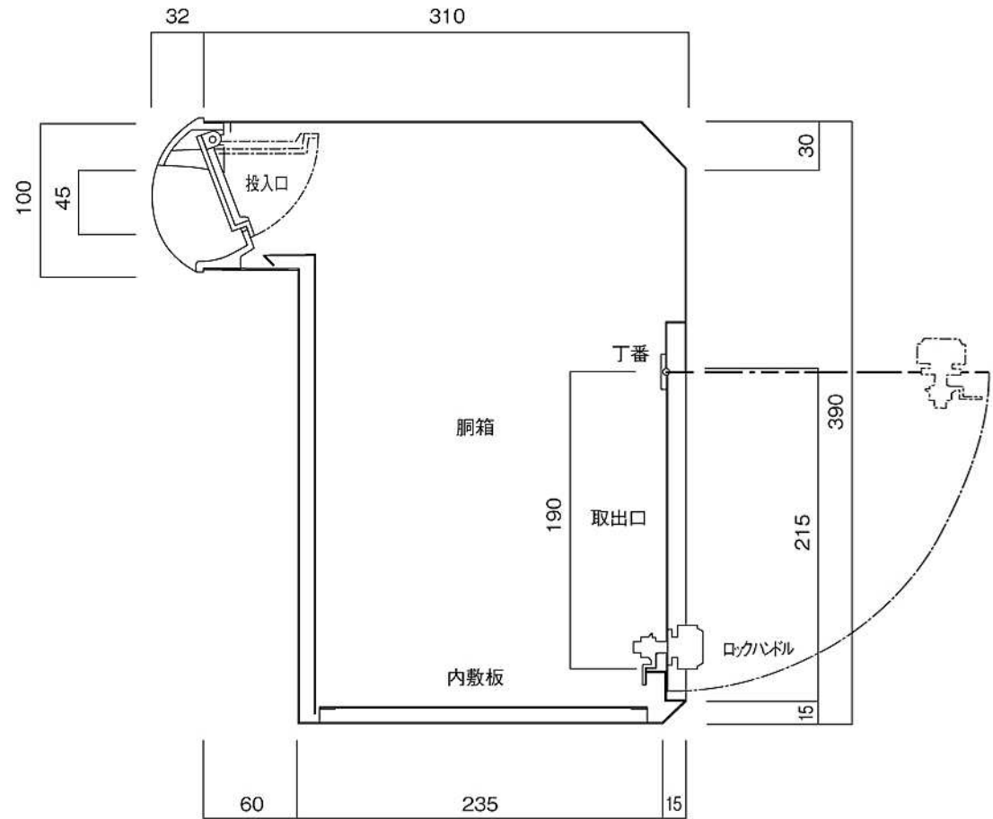
縦断面図
