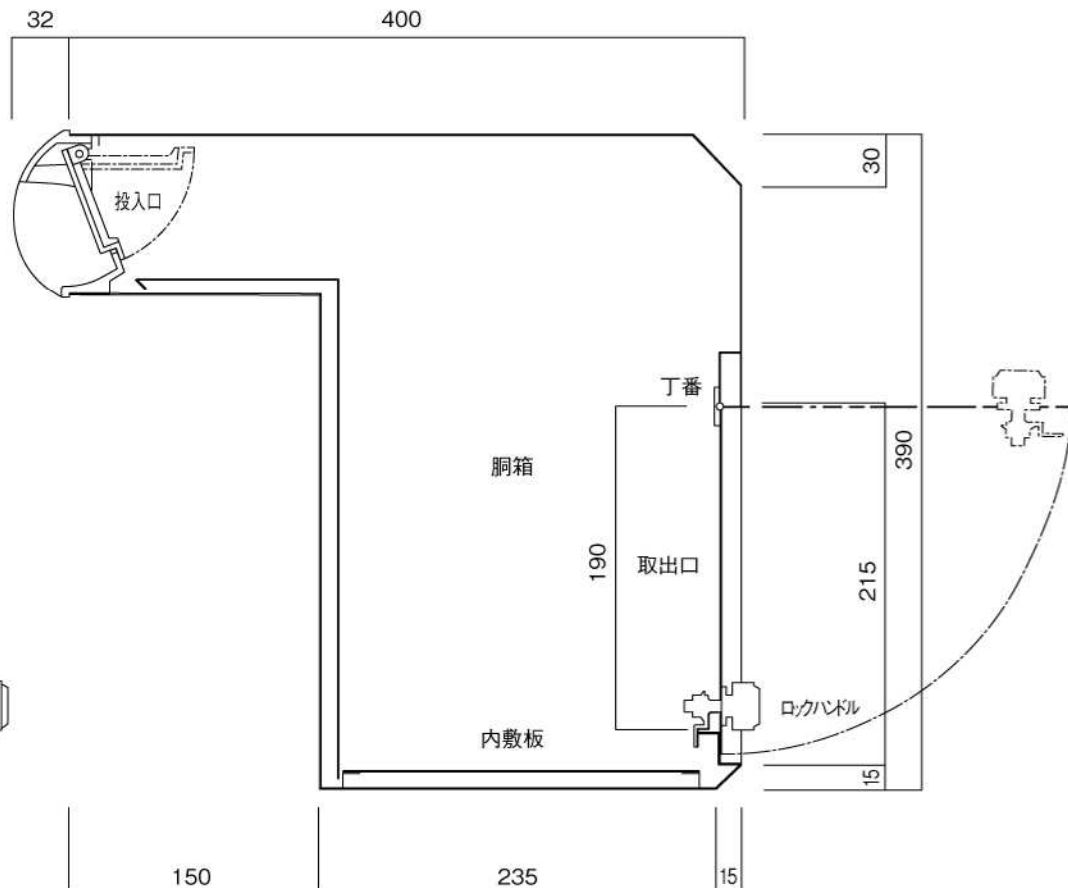
縦断面図
