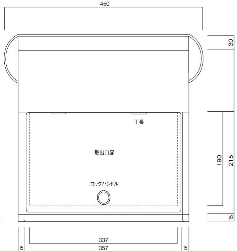
裏面図
