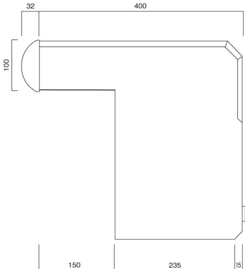
側面図
