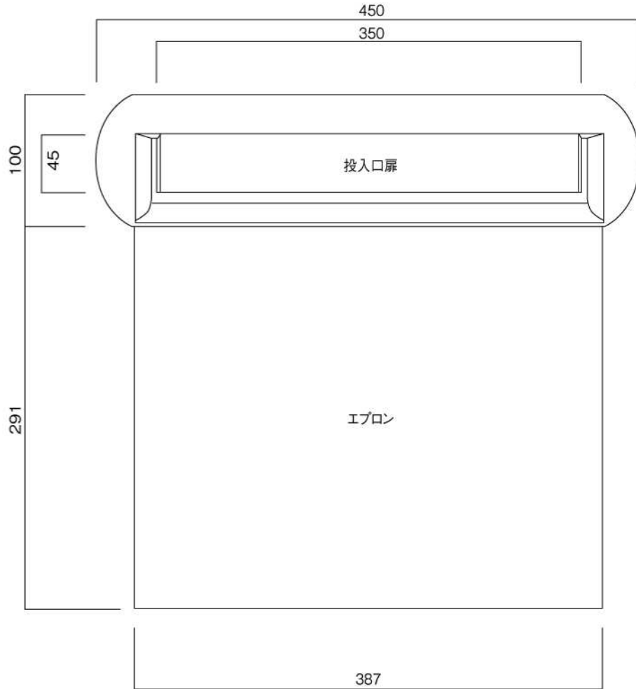
正面図
