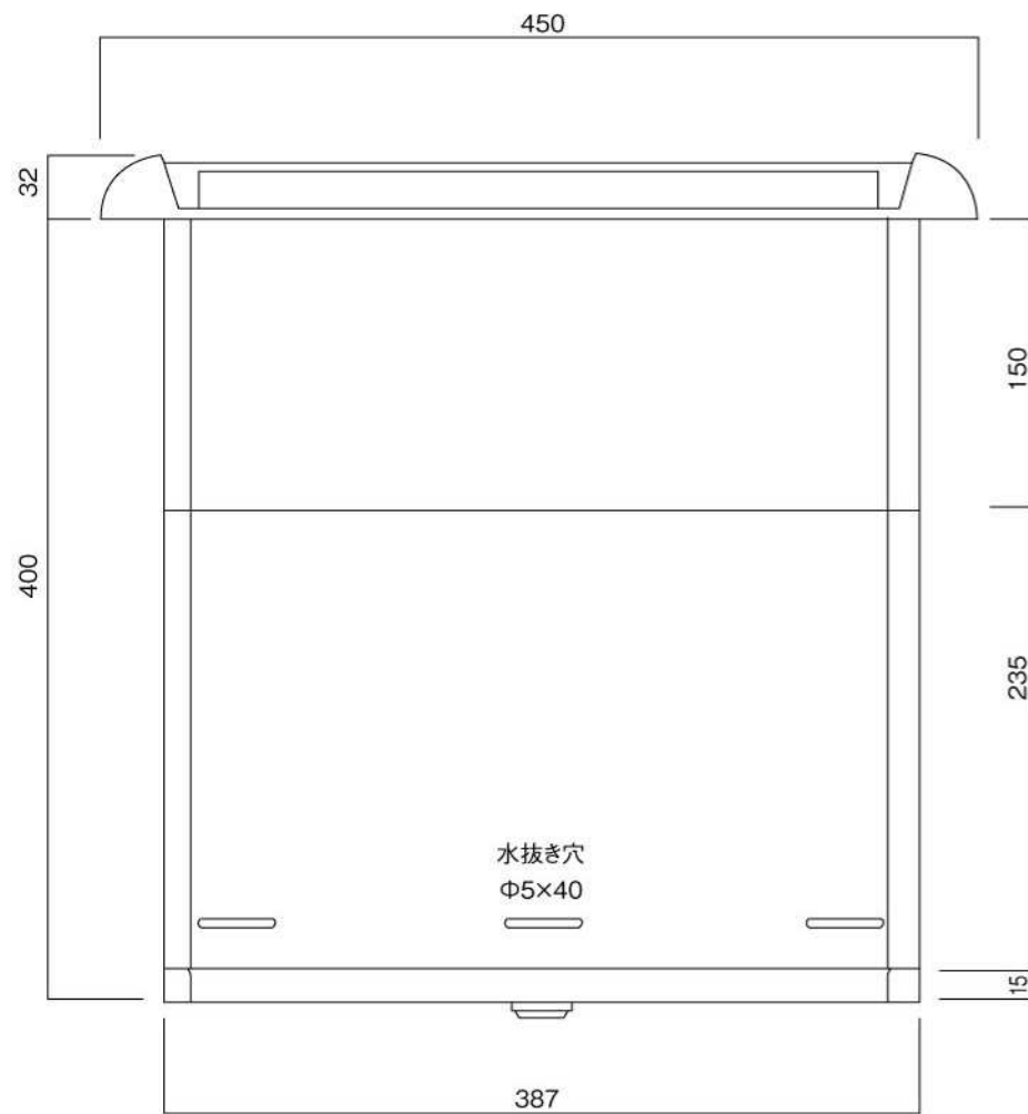
底面図
