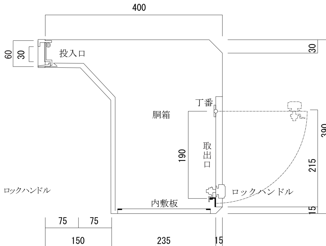
縦断面図
