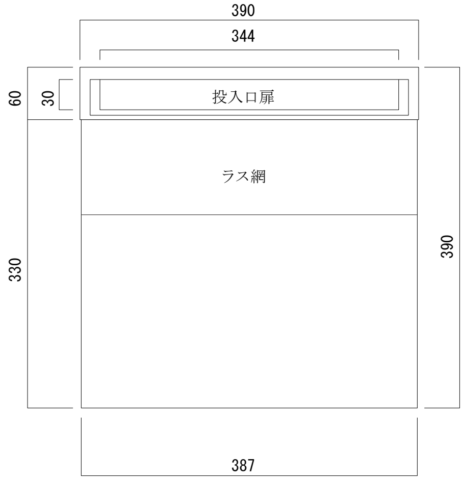
正面図
