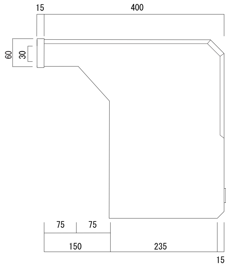
縦断面図
