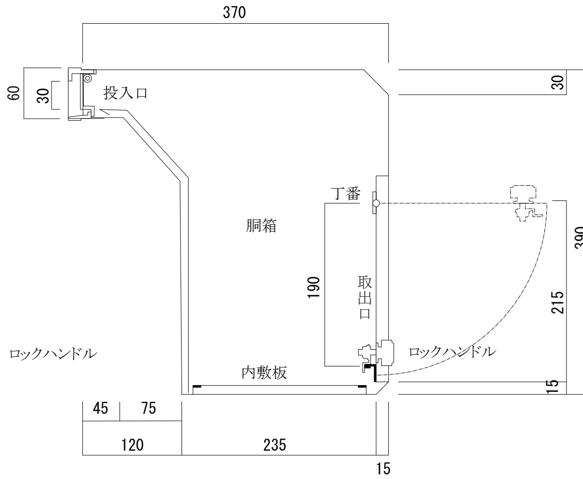
縦断面図
