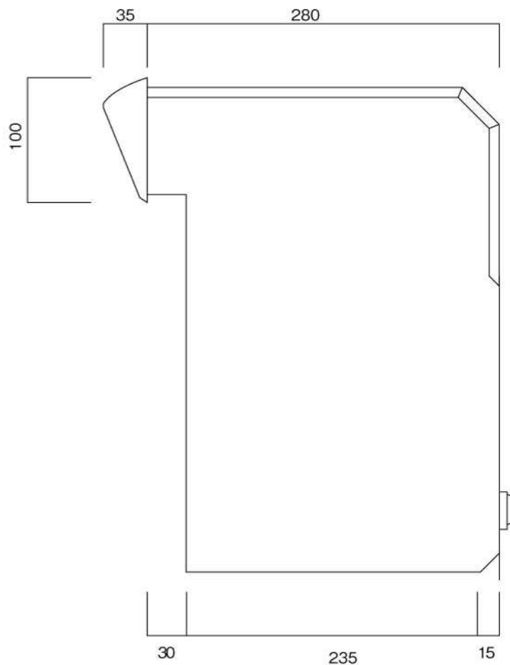
側面図
