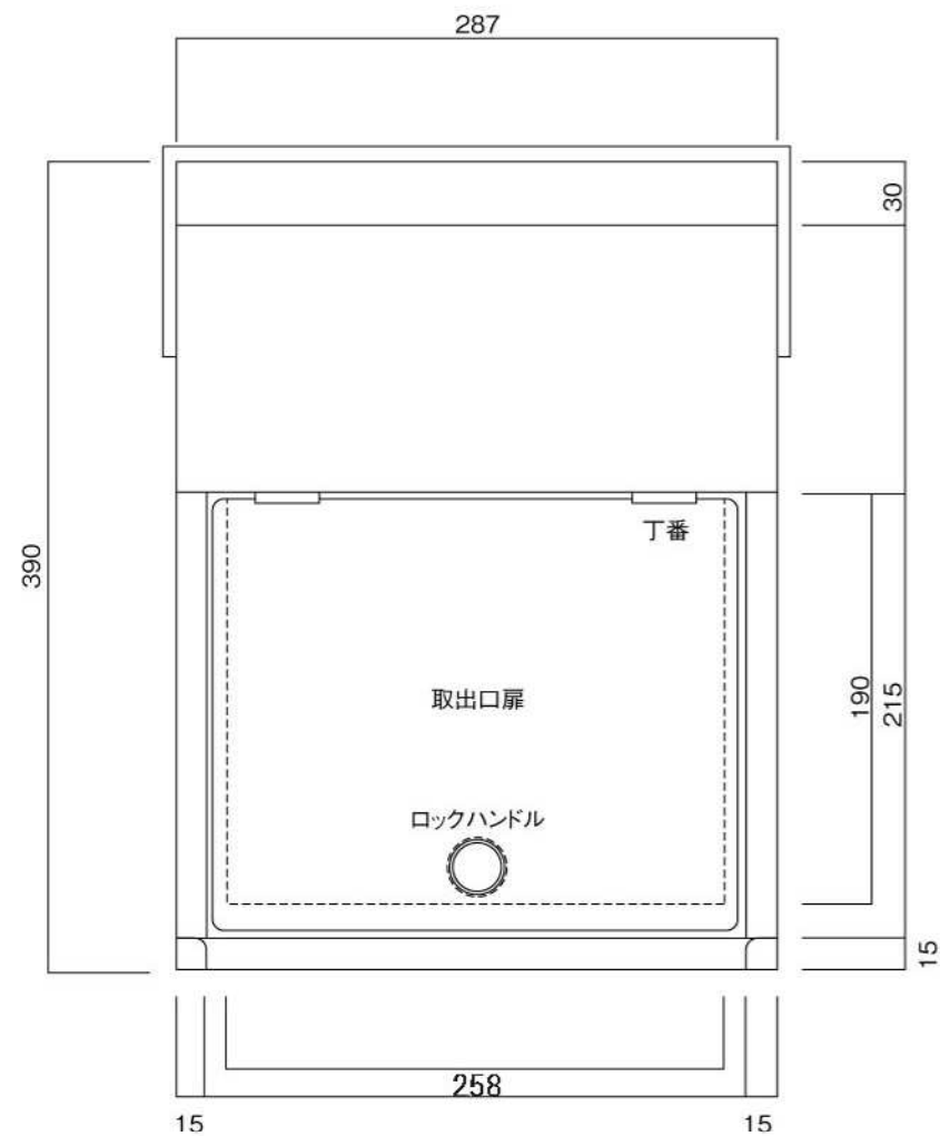
裏面図
