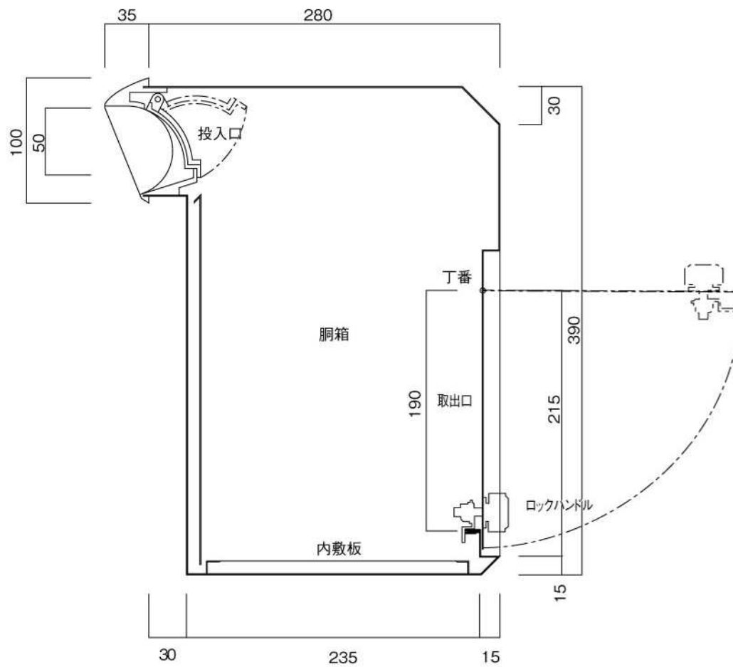
縦断面図
