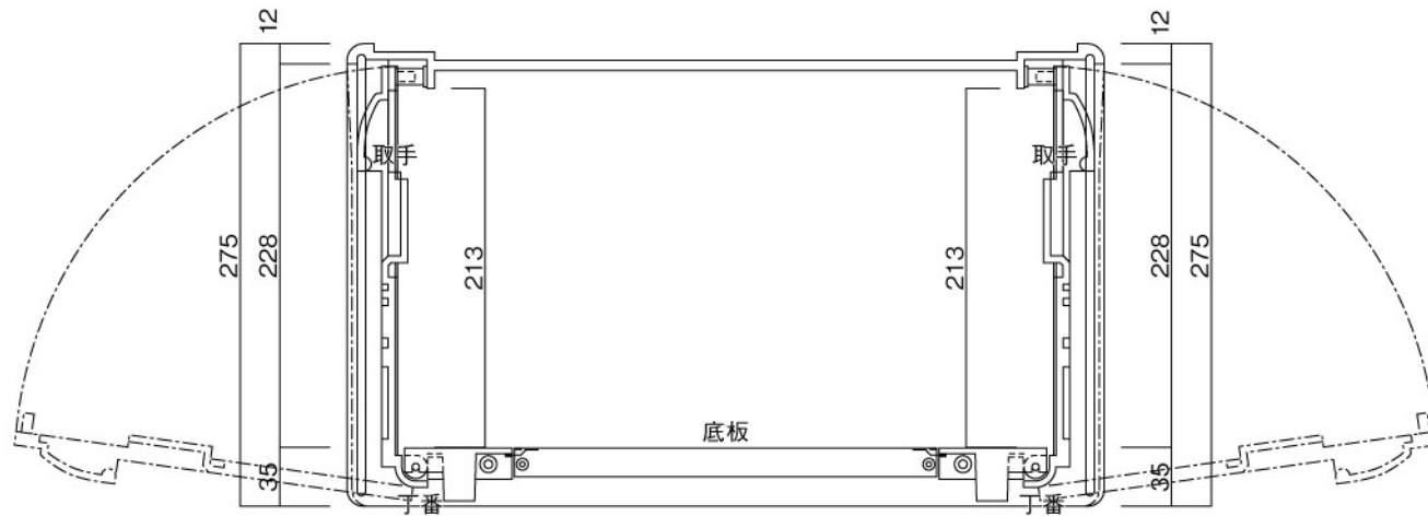
正面図
