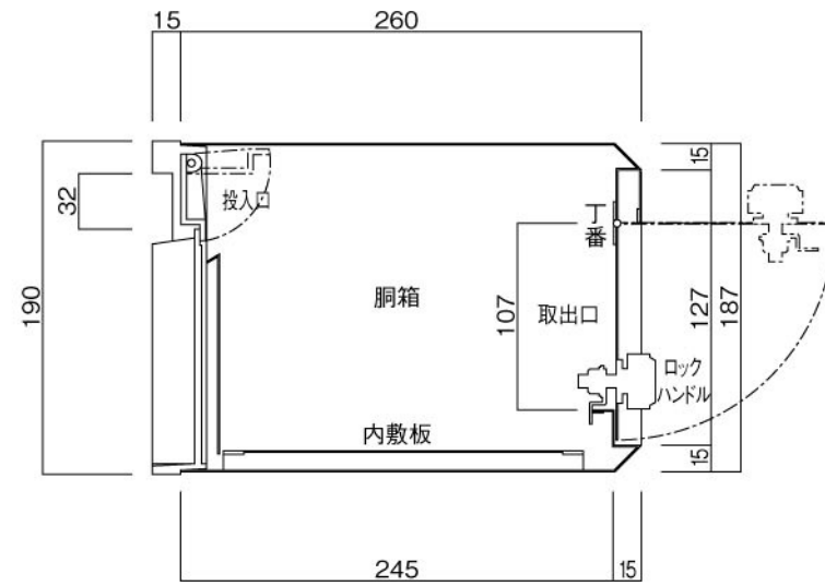
縦断面図
